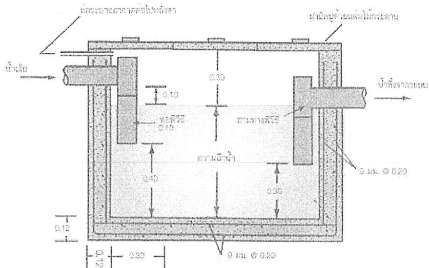
ปอดักไขมันแบบสร้างในที่สำหรับอาคารขนาดใหญ่
